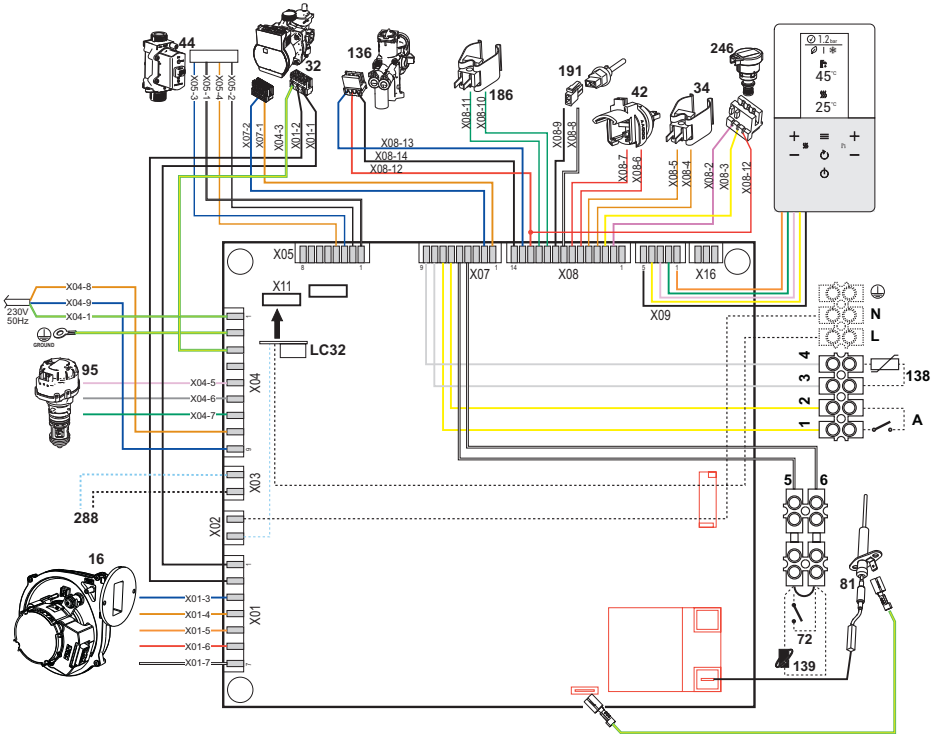
εικ. 81- Ηλεκτρολογικό διάγραμμα
