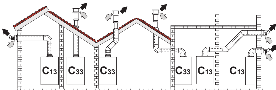
fig. 31 - Esempi di collegamento con tubi coassiali
