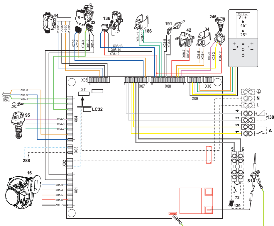
fig. 81 - Schema elettrico
