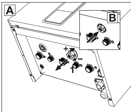
wygląd 26- Pokrętło napełniania
