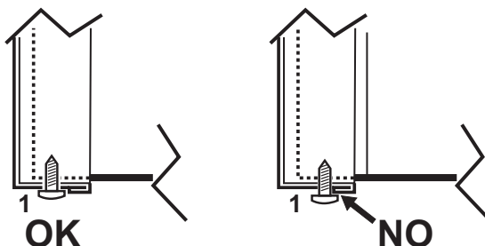
fig. 57- Posición correcta del panel frontal
