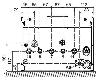
wygląd 76- Widok z dołu
