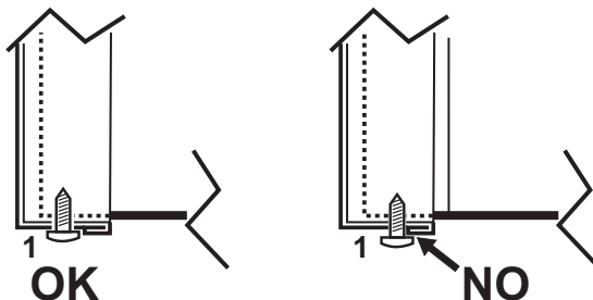
εικ. 57- Σωστή τοποθέτηση μπροστινού πίνακα
