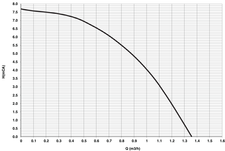
fig. 80 - Carga hidrostática residual disponible en la instalación
