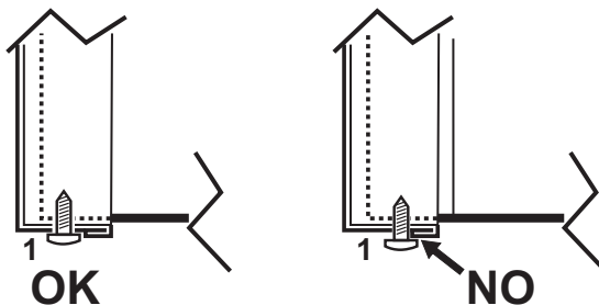
wygląd 57- Prawidłowe położenie przedniego panelu
