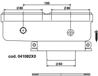
wygląd 36- Człon początkowy do montażu oddzielnych przewodów
