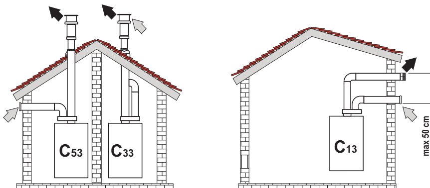
fig. 35 - Esempi di collegamento con tubi separati
