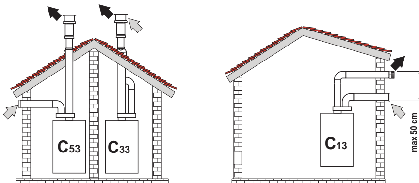
fig. 35- Exemple de racordare cu tuburi separate
