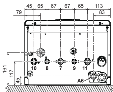
fig. 76- Vista inferior
