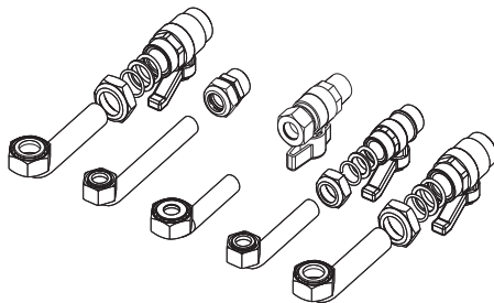
fig. 28 - Kit idraulico
