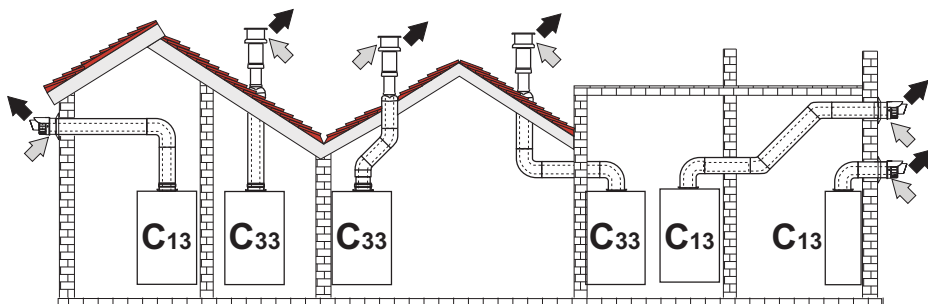
fig. 31- Ejemplos de conexión con tubos coaxiales
