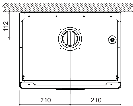
fig. 75- Vista superior
