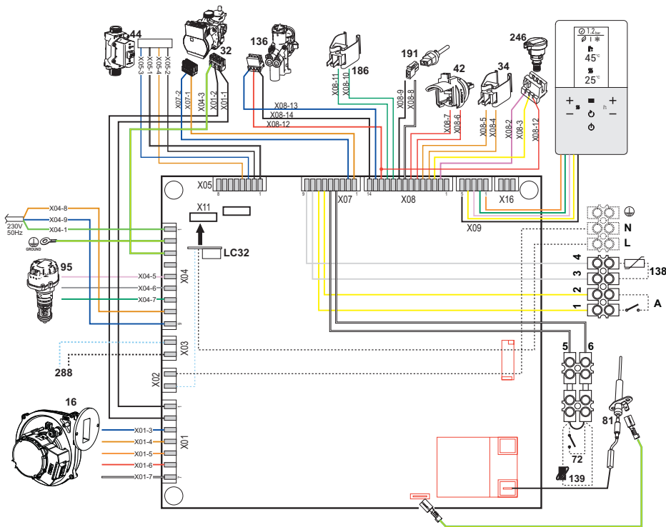
wygląd 81 - Schemat instalacji elektrycznej
