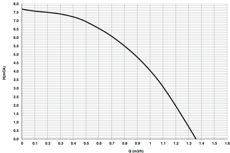
wygląd 80- Wysokość podnoszenia dostępna dla układu
