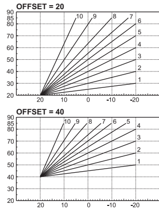
εικ. 25- Παράδειγμα παράλληλης μετατόπισης των καμπυλών αντιστάθμισης
