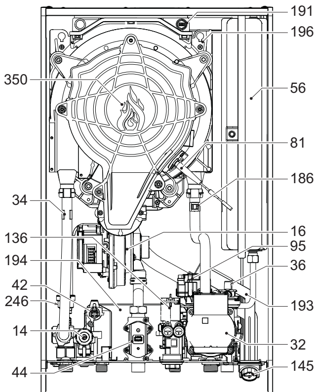
fig. 77 - Vista generale
