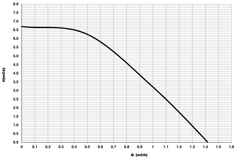
fig. 79 - Prevalenza residua disponibile all'impianto
