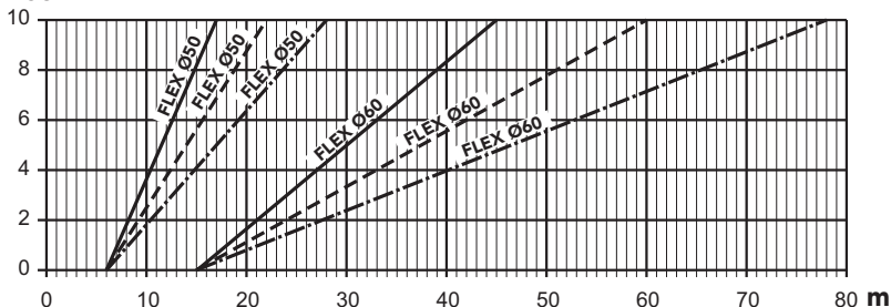
wygląd 40- Wykres wyboru parametrów przewodu spalinowego
