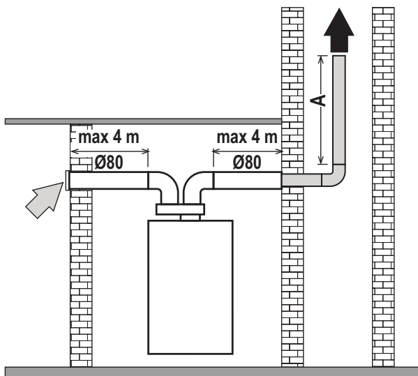
fig. 39 - Schema per solo intubamento con tubo flessibile
