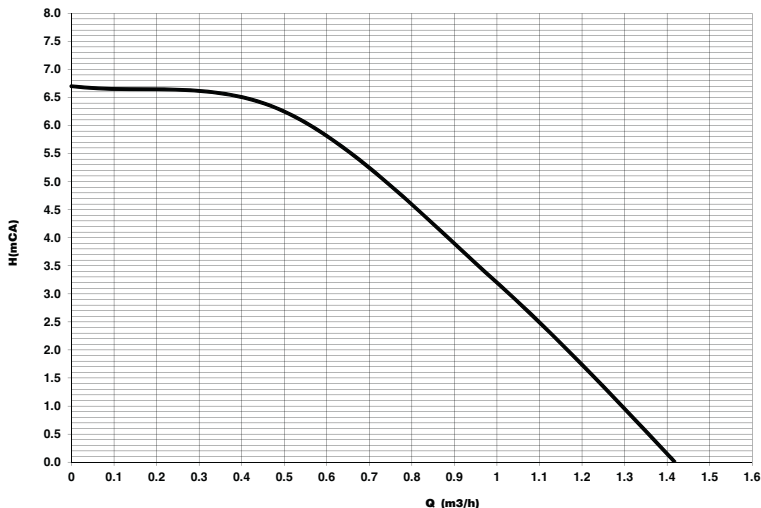
εικ. 79- Διαθέσιμο υπολειπόμενο μανομετρικό ύψος στην εγκατάσταση
