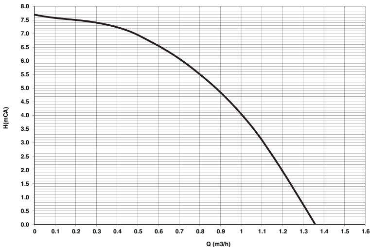
εικ. 80- Διαθέσιμο υπολειπόμενο μανομετρικό ύψος στην εγκατάσταση
