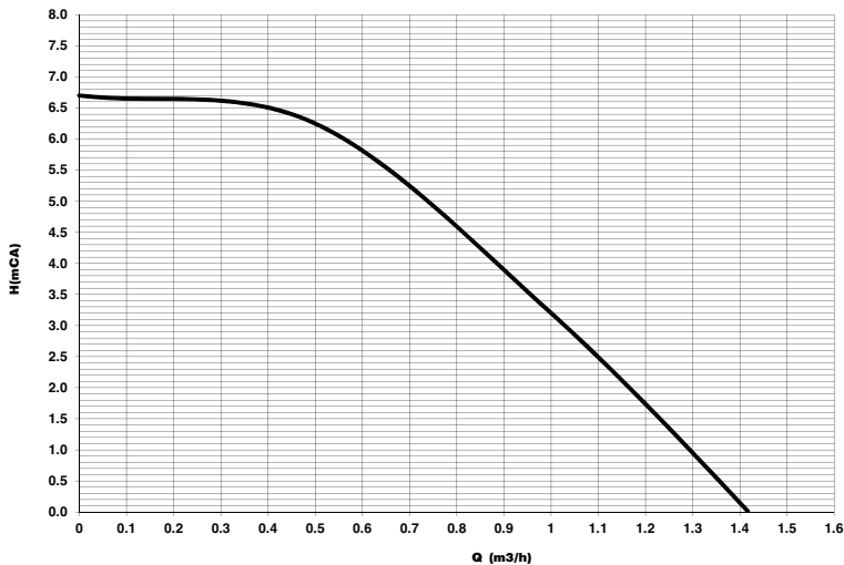
fig. 79 - Carga hidrostática residual disponible en la instalación
