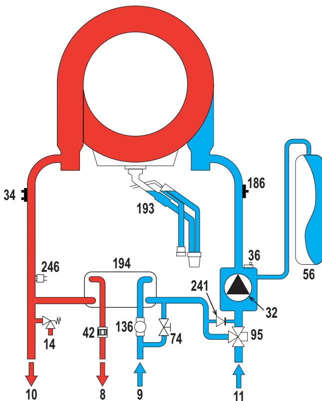
fig. 78- Circuito hidráulico
