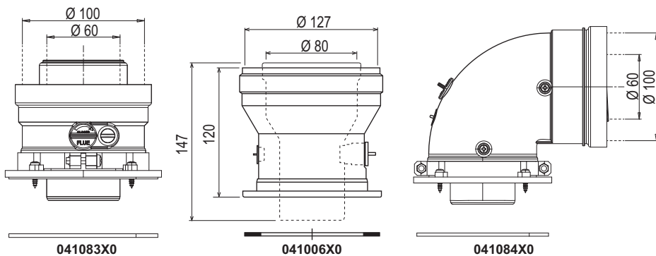
fig. 32- Accesorios iniciales para conductos coaxiales
