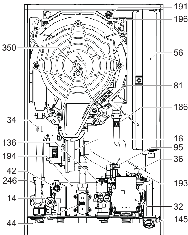
wygląd 77- Widok ogólny
