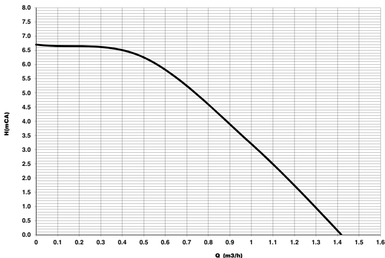
wygląd 79- Wysokość podnoszenia dostępna dla układu
