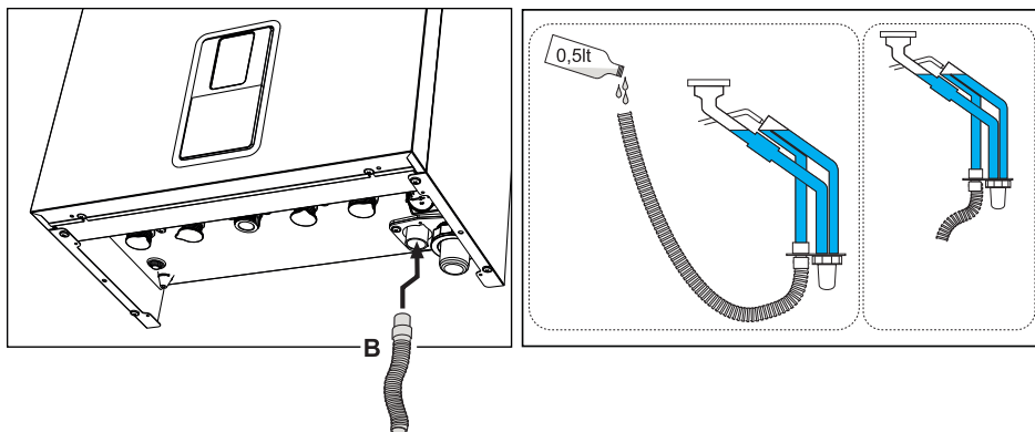
fig. 52- Conexión de la descarga de condensado
