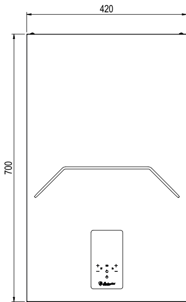
wygląd 73- Widok z przodu
