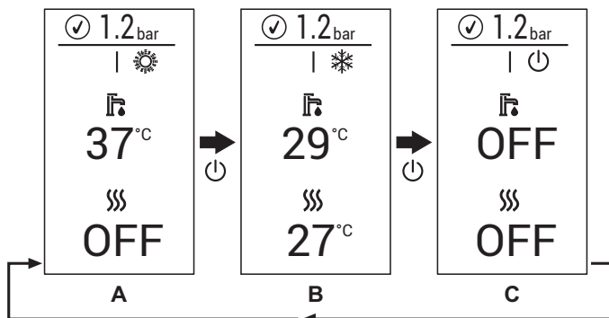
fig. 11 - Spegnimento caldaia
