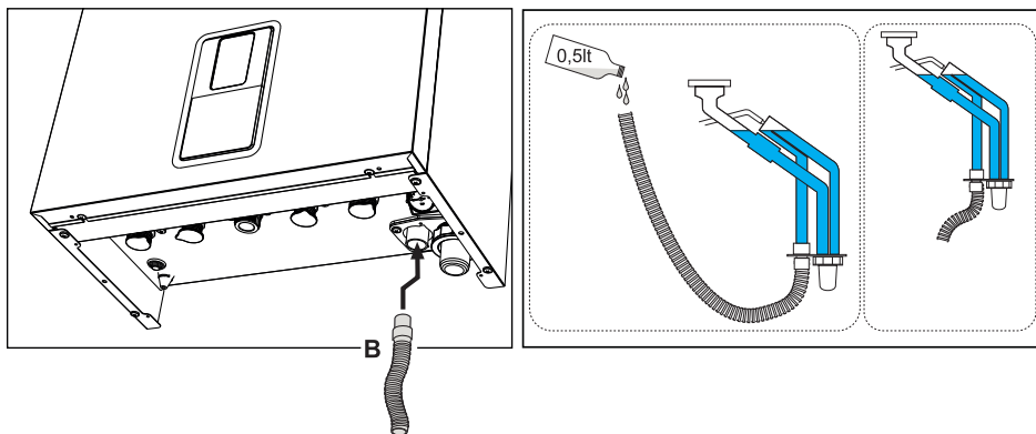
wygląd 52- Podłączenie spustu kondensatu
