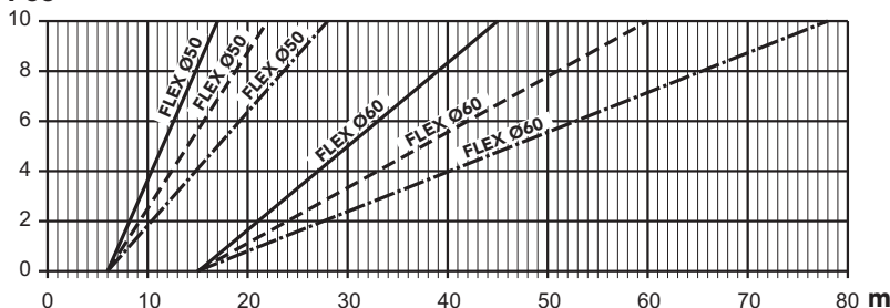
fig. 40- Chart for flue parameter choice
