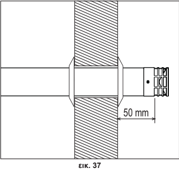
Απόσταση απόληξης (Τύπος C13)
