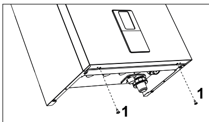
wygląd 56- Otwieranie panelu przedniego
