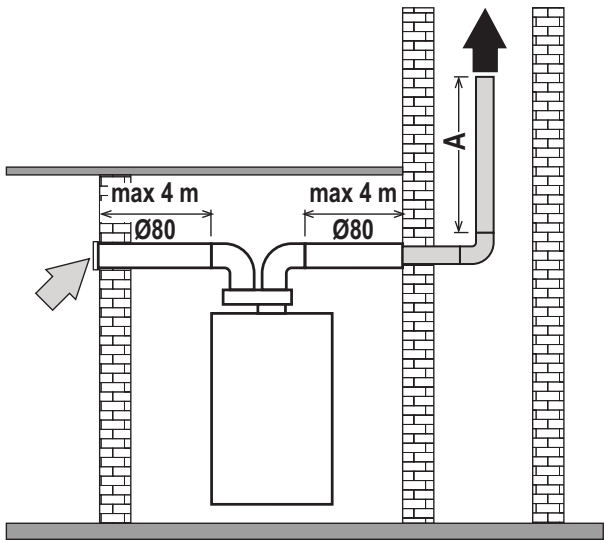
fig. 39- Esquema solo para entubamiento con flexible
