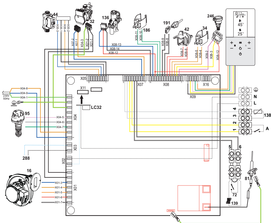
fig. 81 - Esquema eléctrico
