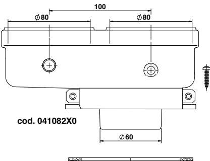
fig. 36- Accesorio inicial para conductos separados
