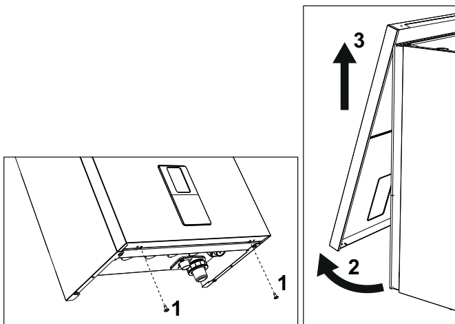
fig. 56 - Apertura pannello frontale
