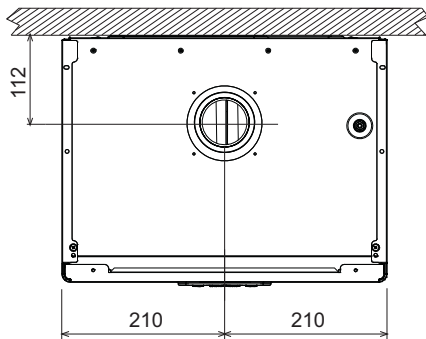
wygląd 75- Widok z góry
