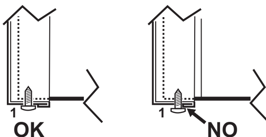
fig. 57 - Posizione corretta pannello frontale
