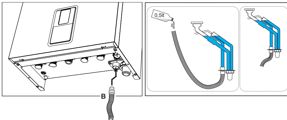
fig. 52 - Collegamento scarico condensa
