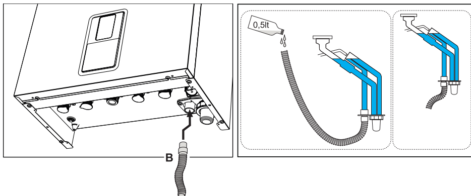
ΕΙΚ. 52- Σύνδεση εξαγωγής συμπυκνώματος
