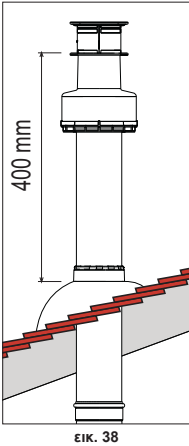
Απόσταση απόληξης (Τύπος C33)
