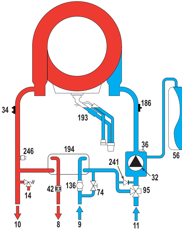
εικ. 78- Υδραυλικό κύκλωμα
