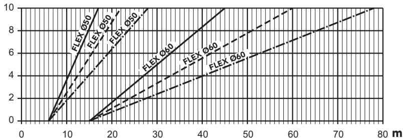
fig. 40- Grafic pentru alegerea parametrului pentru horn
