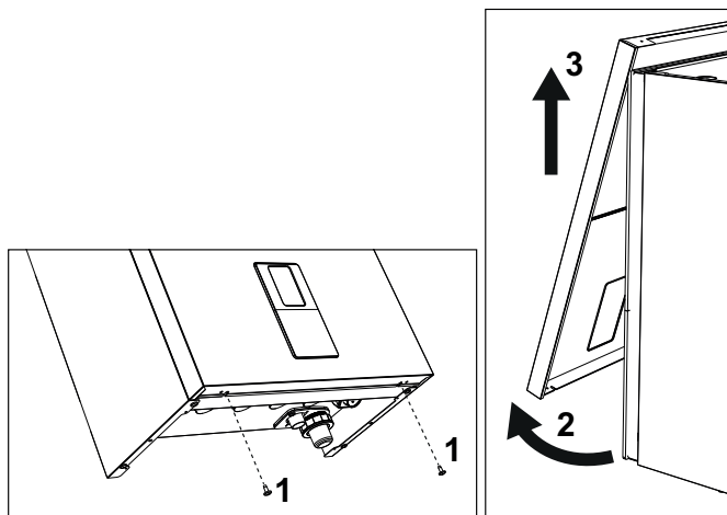
fig. 56- Apertura del panel frontal
