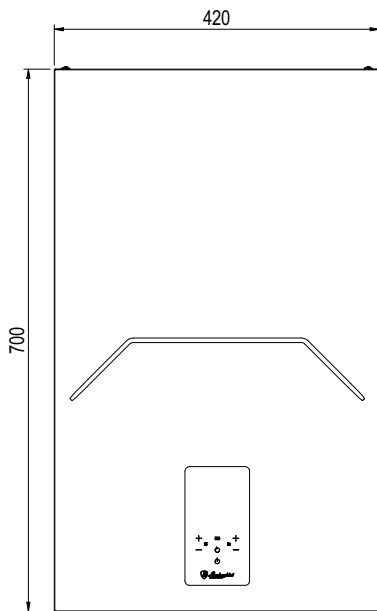
εικ. 73- Μπροστινή όψη
