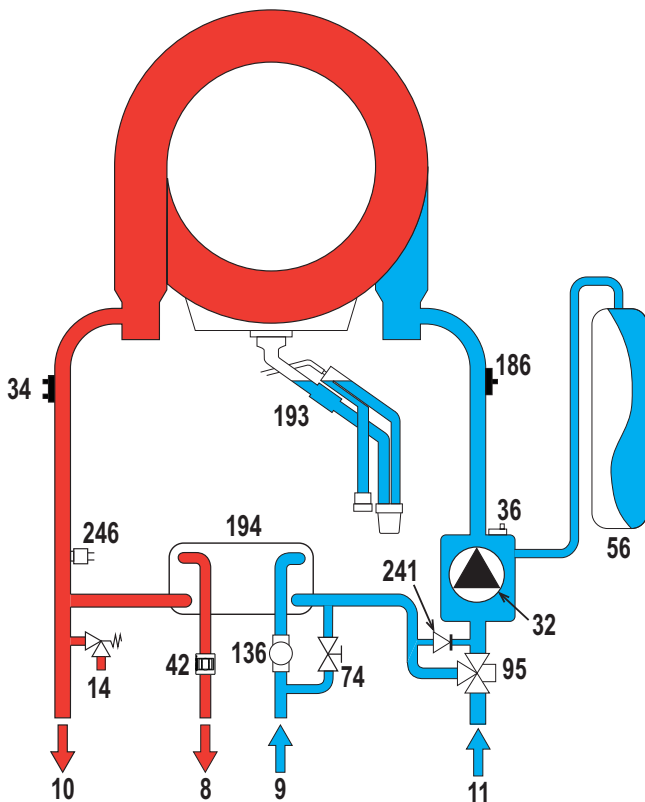
wygląd 78- Obieg wody
