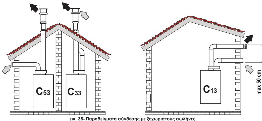
εικ. 35- Παραδείγματα σύνδεσης με ξεχωριστούς σωλήνες
