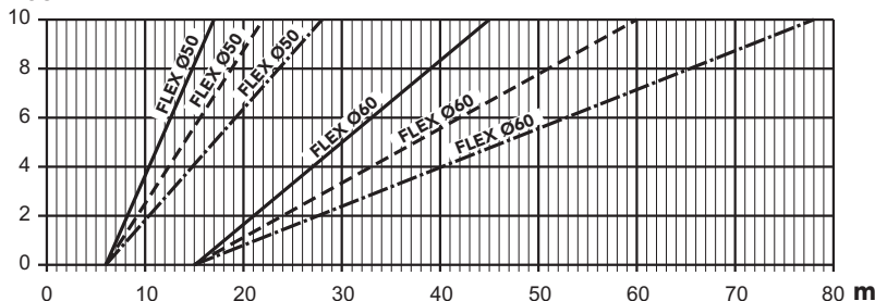
fig. 40- Gráfico para seleccionar el parámetro chimenea
