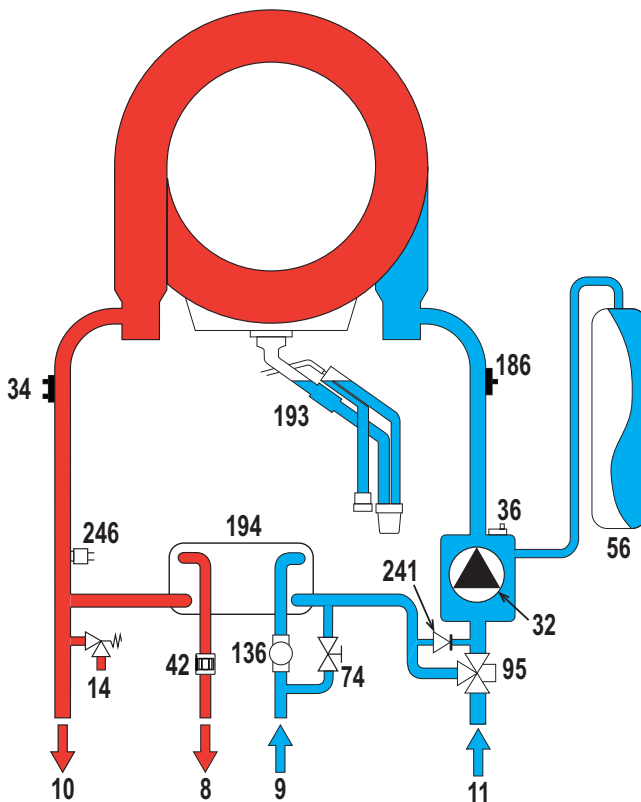
fig. 78 - Circuito idraulico
