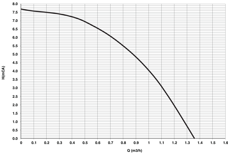
fig. 80 - Prevalenza residua disponibile all'impianto
