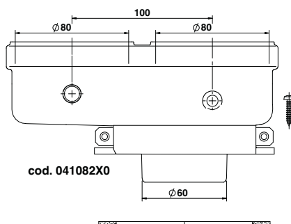
fig. 36 - Accessorio di partenza per condotti separati
